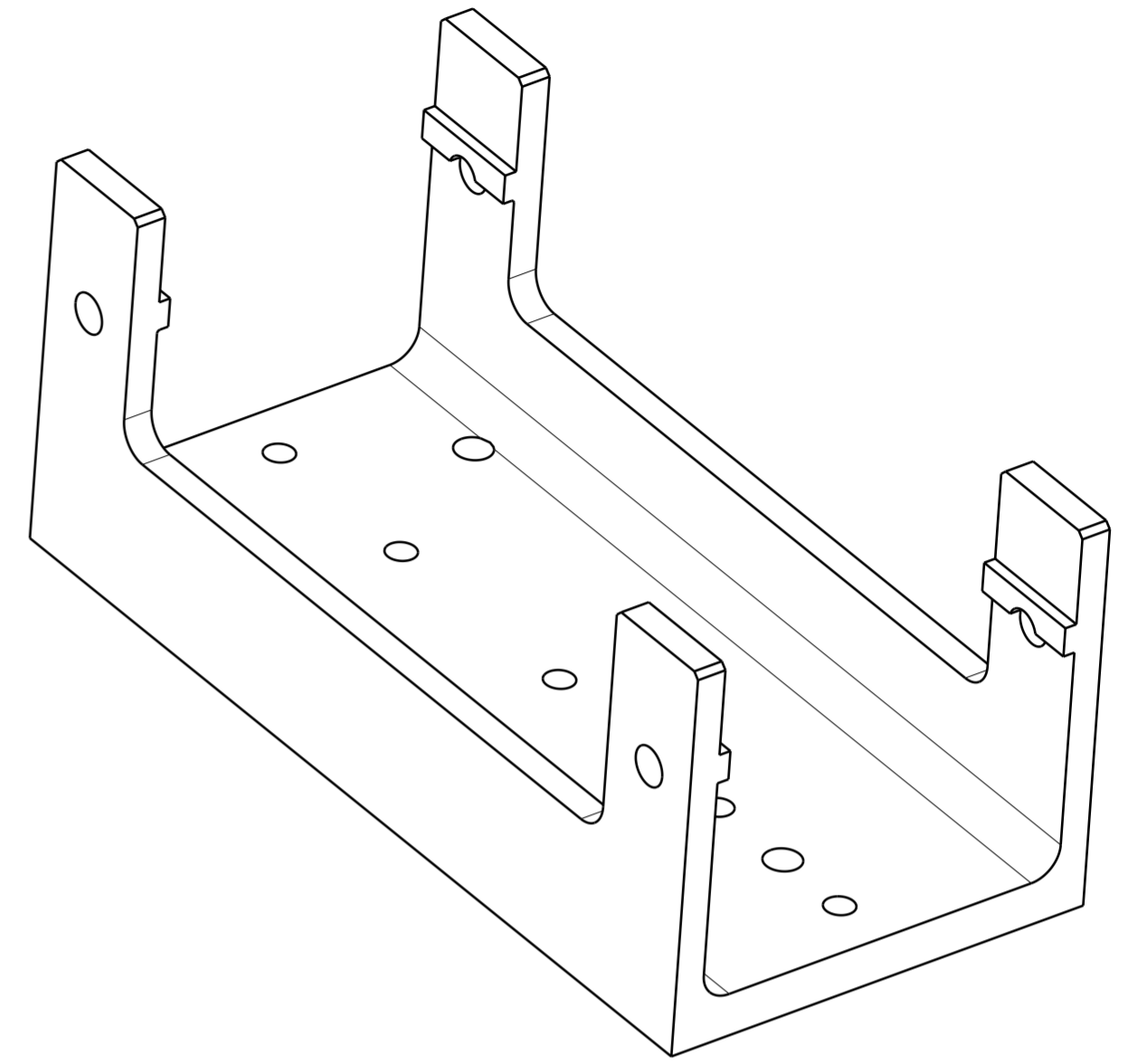
Isometric view Scale: 1:1
