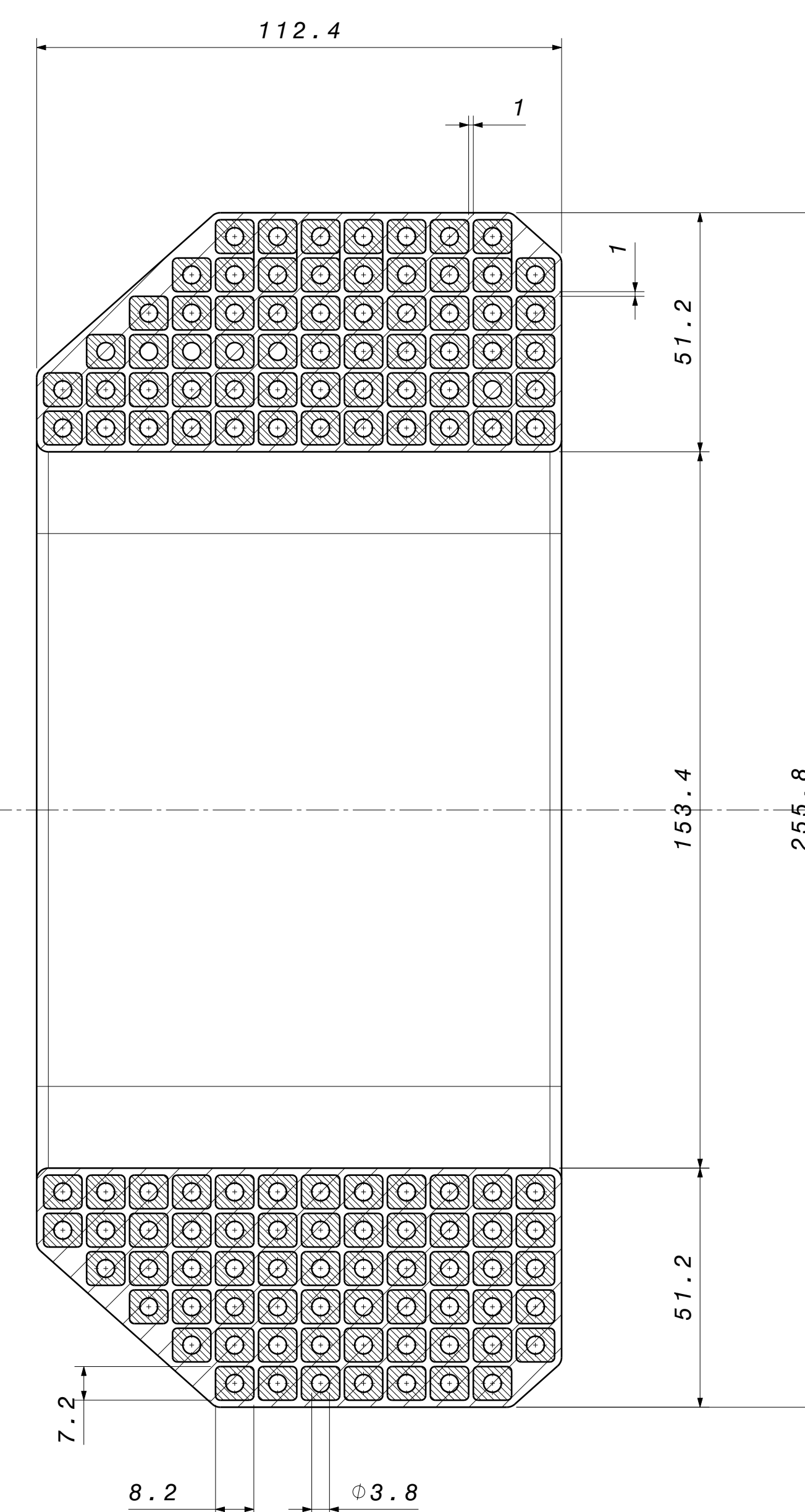
Section view A-A Scale: 1:1
