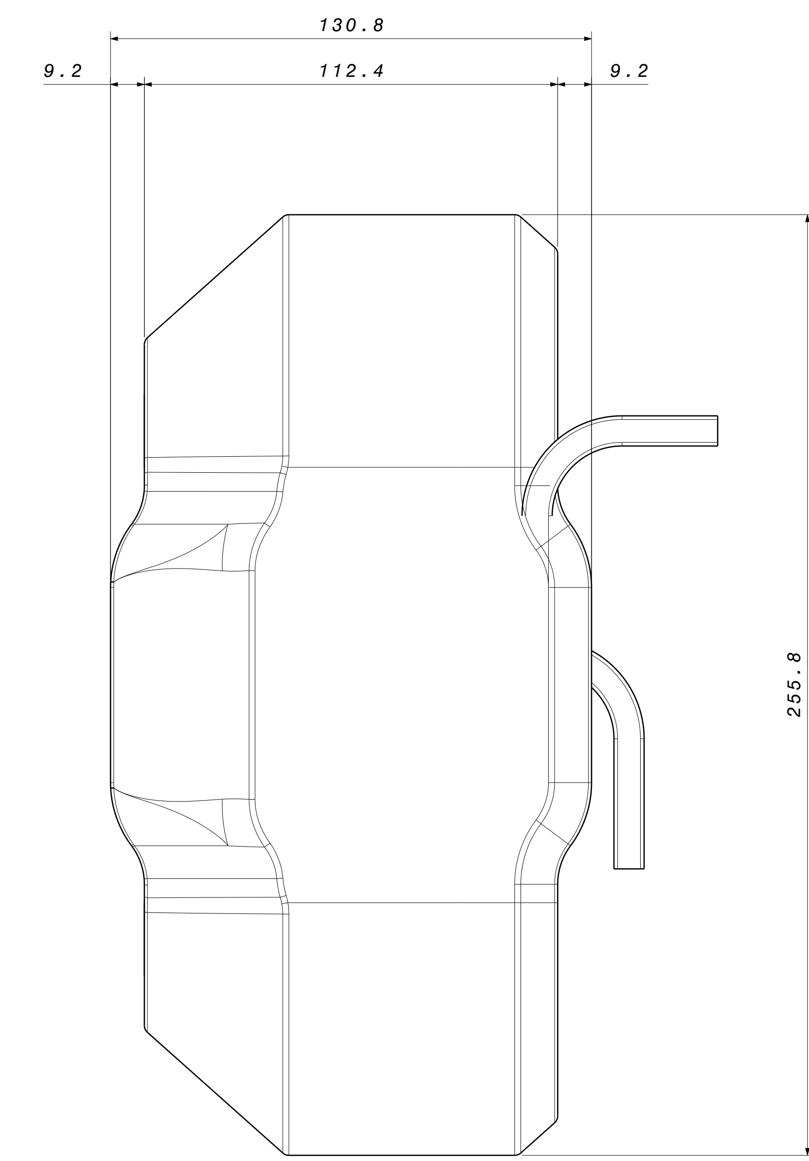
Left view Scale: 1:1
