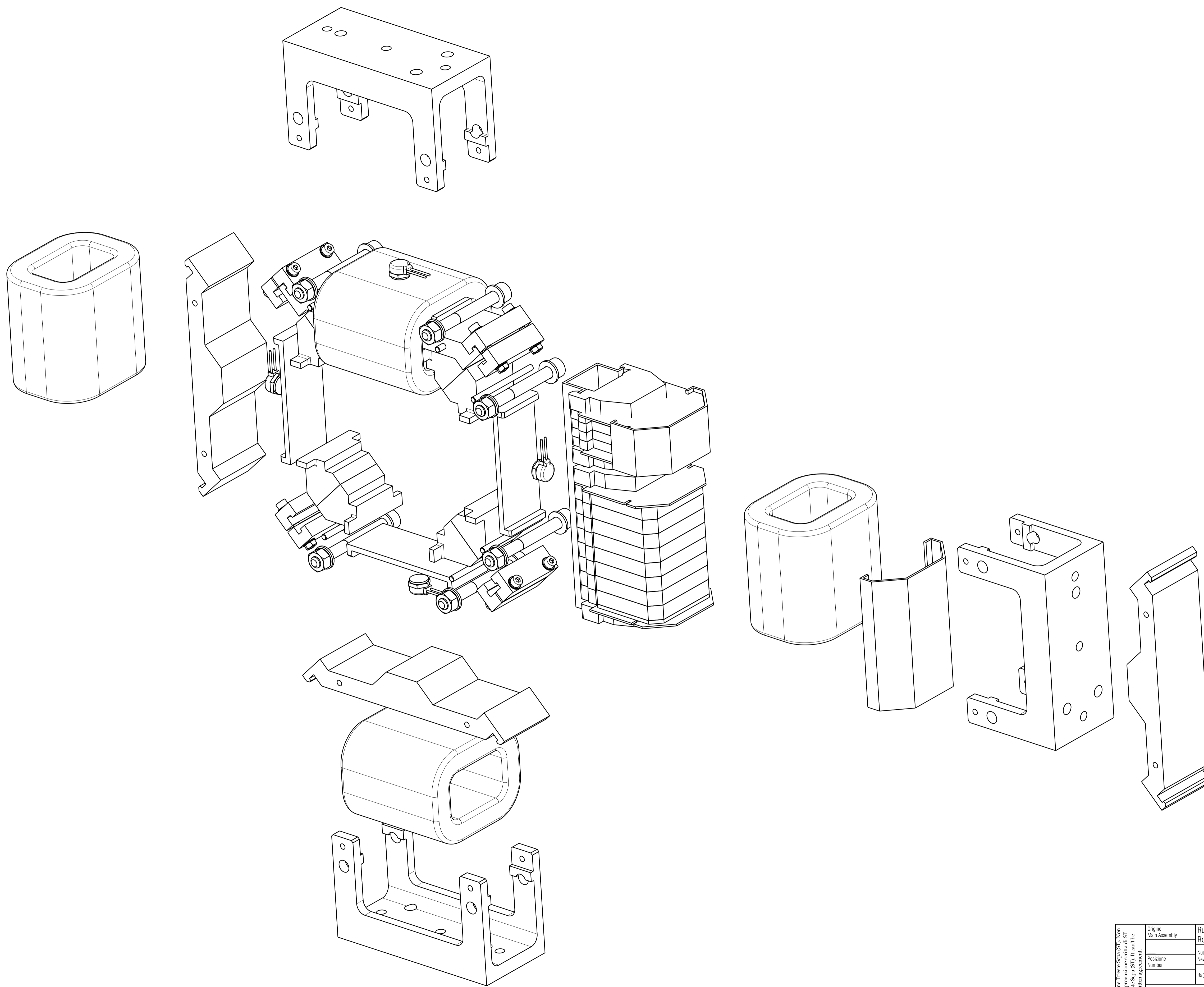
Isometric view Scale: 1:1
